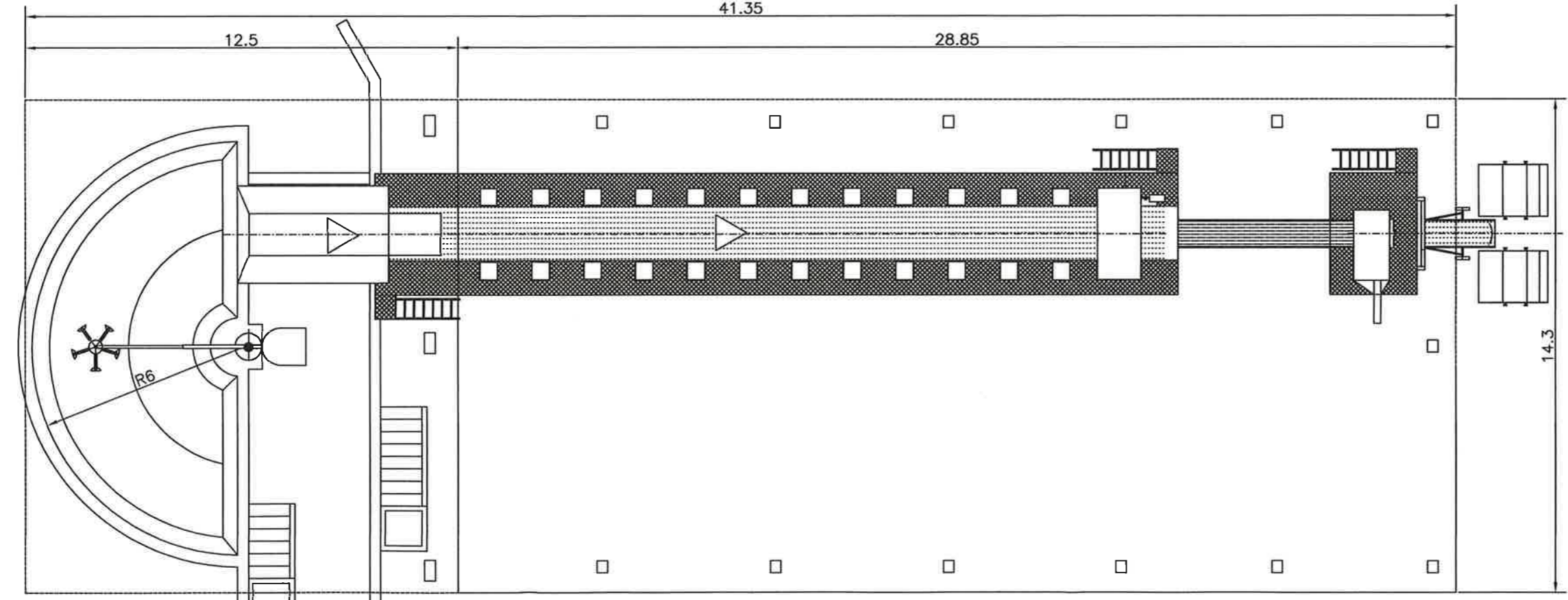
PLANTA
